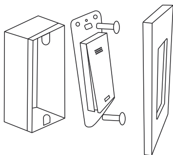
Instalação de embutir
